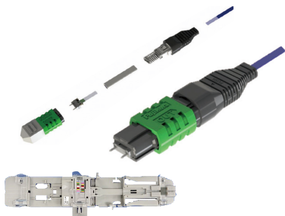
単心集合工具 (RT-02)
